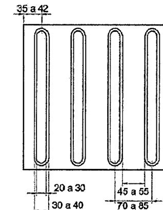
Sinalização tátil direcional – Modulação do piso (dimensões em mm)
