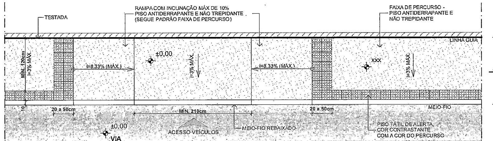
Figura 5 – Solução para acesso de veículos em calçada com largura do passeio não suficiente para acomodar o rebaixamento e a faixa de percurso com largura de no mínimo 1,20 m
