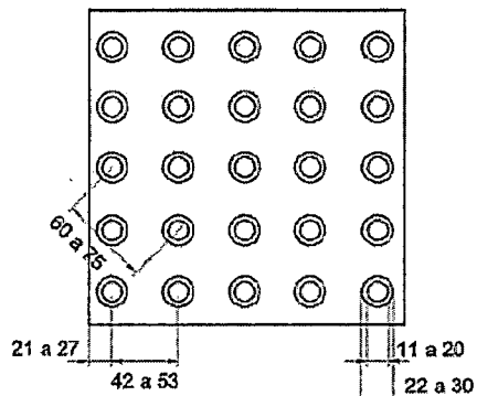
Sinalização tátil de alerta – Modulação do piso (dimensões em mm)
