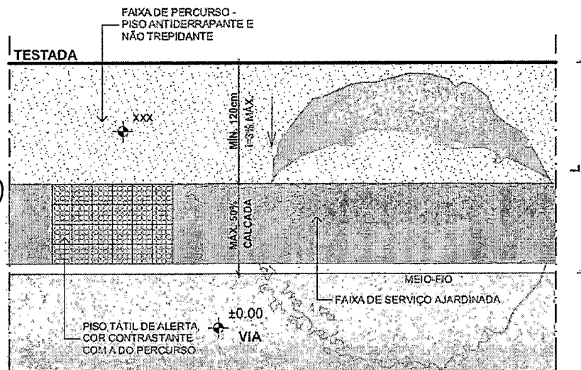
Figura 6 - Calçada com 01 faixa ajardinada
