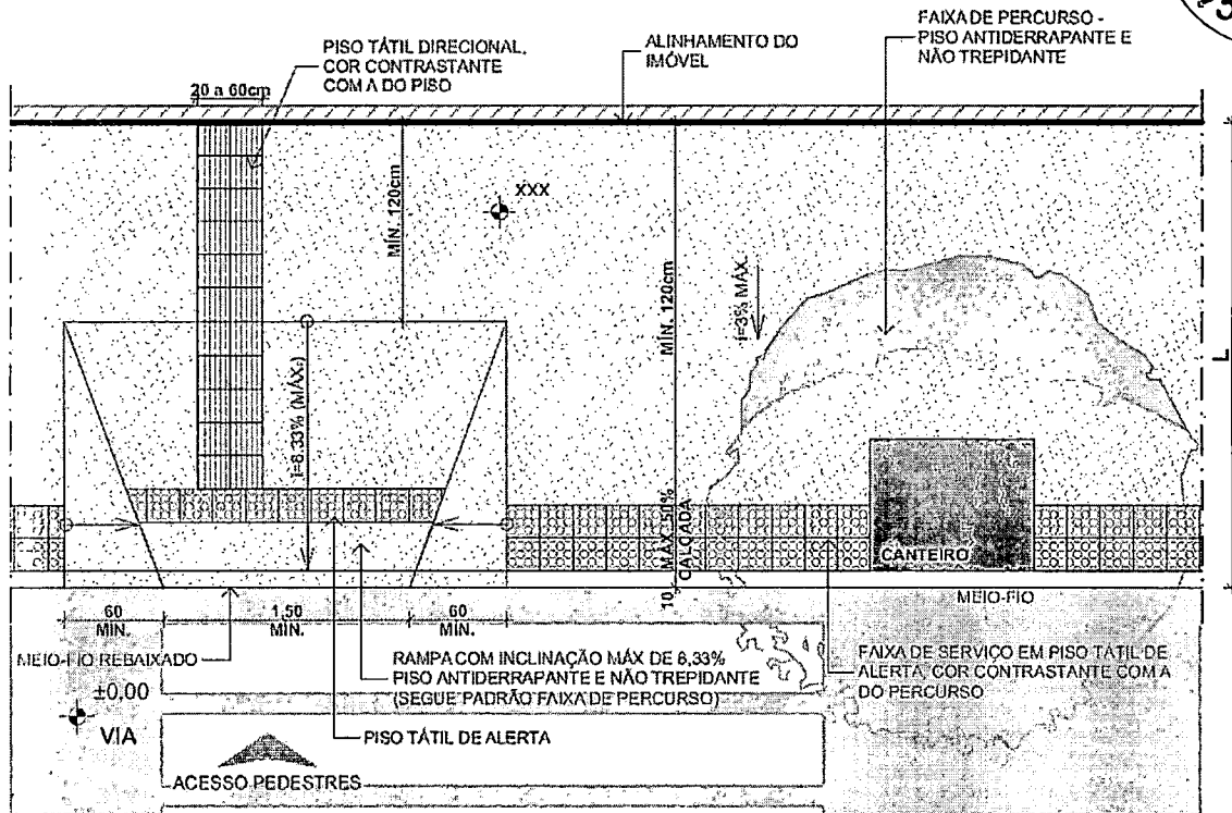
Figura 9 -- Rebaixamento de meio-fio com rampa de acesso de pedestres em calçada com 02 faixas diferenciadas
