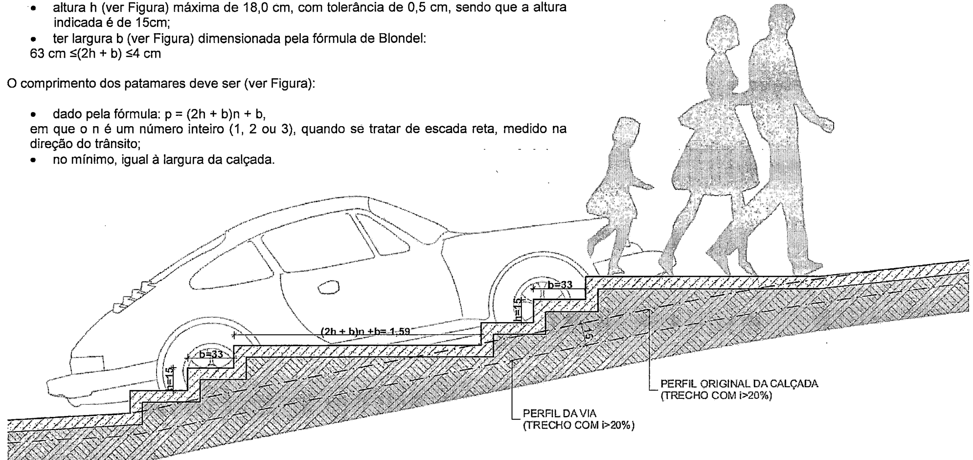
Figura 7 - Corte longitudinal de calçada em via de declividade superior a 20% - exemplo
